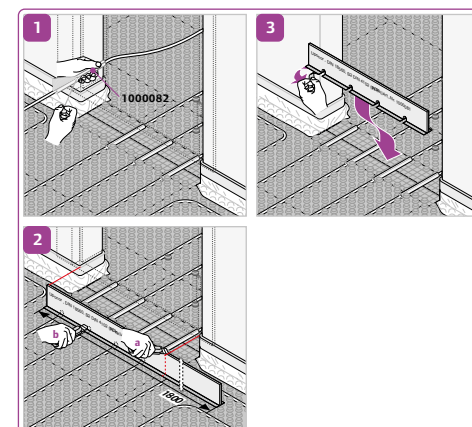
Монтаж компенсационного элемента с использованием фольги под 45°
