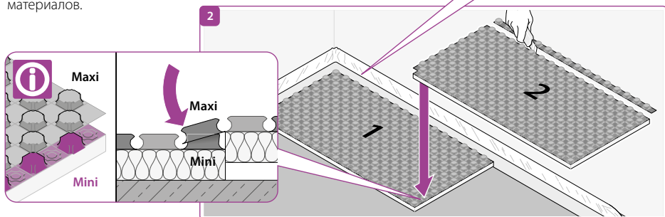
Укладка панелей
